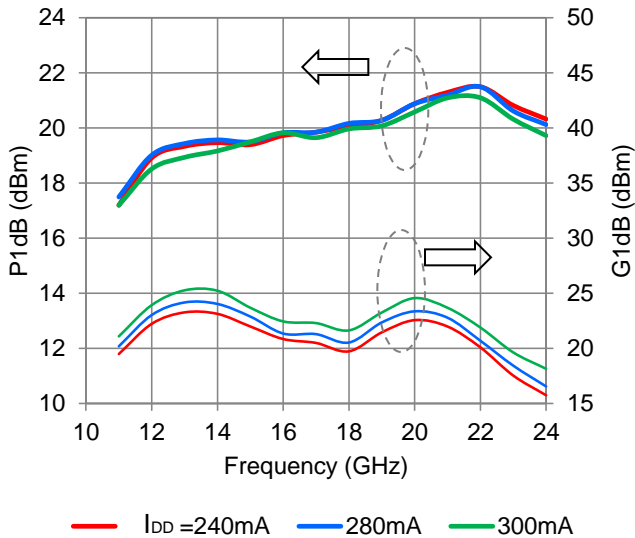
P1dB, G1dB vs. I DD
